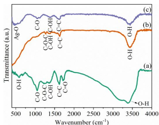
Fig. 2. FTIR spectra of a) rGO, b) \text{Ag}_2\text{O} , and c) \text{rGO@Ag}_2\text{O}
